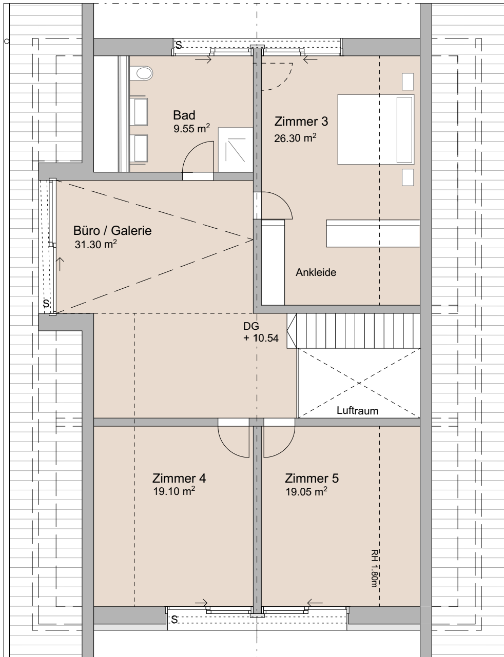
■ W3_ Maisonette 2.OG /DG 7.5 Zi Whg Nettowoohnfläche 235.80 m 2
