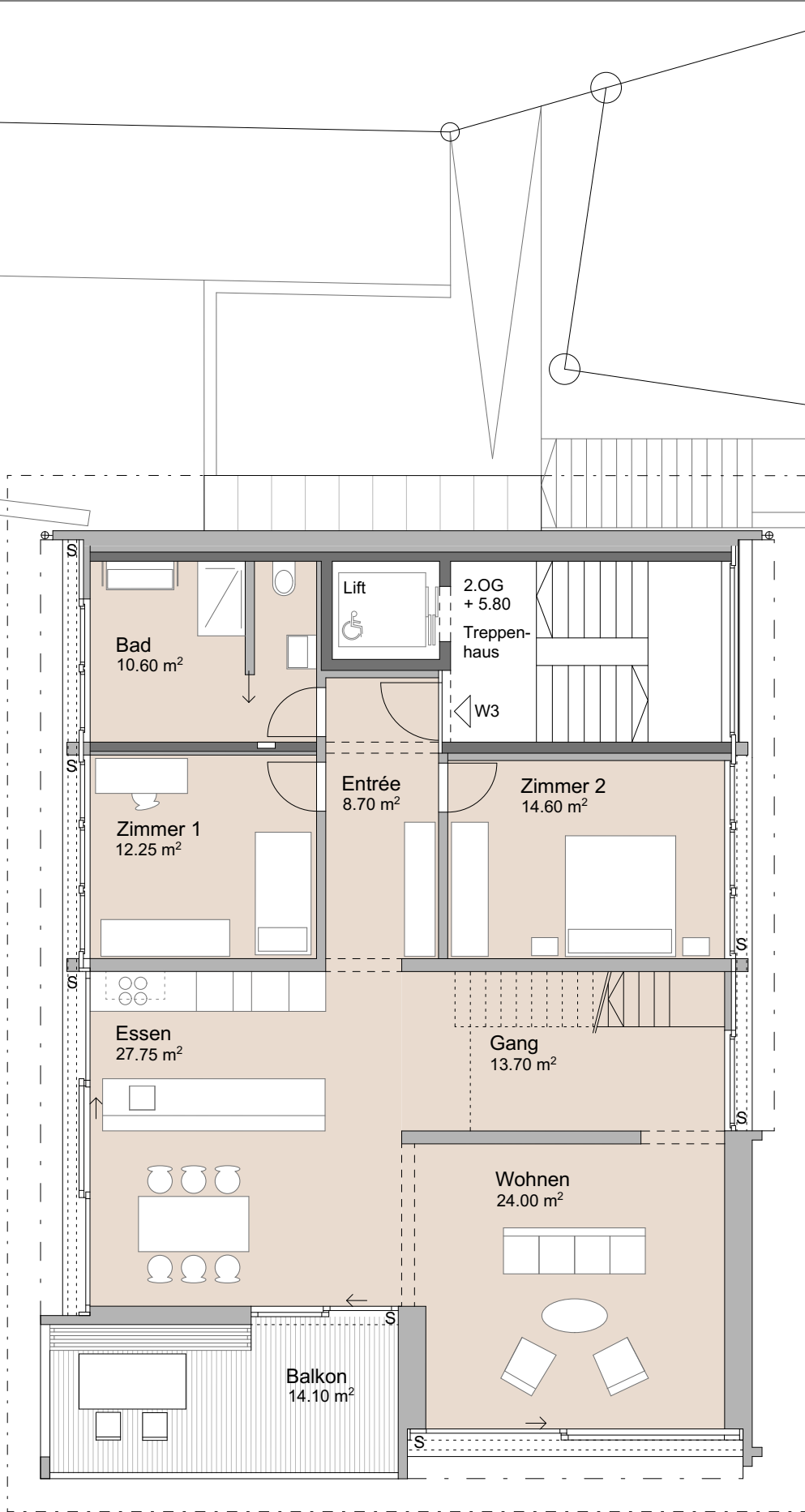
■ W3_ Maisonette 2.OG /DG 7.5 Zi Whg Nettowofläche 235.80 m 2
