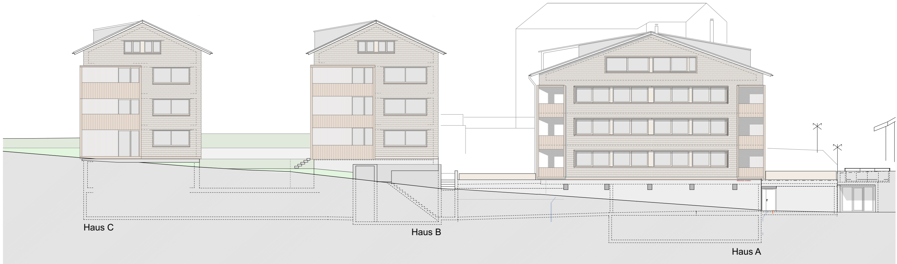
Südfassade
