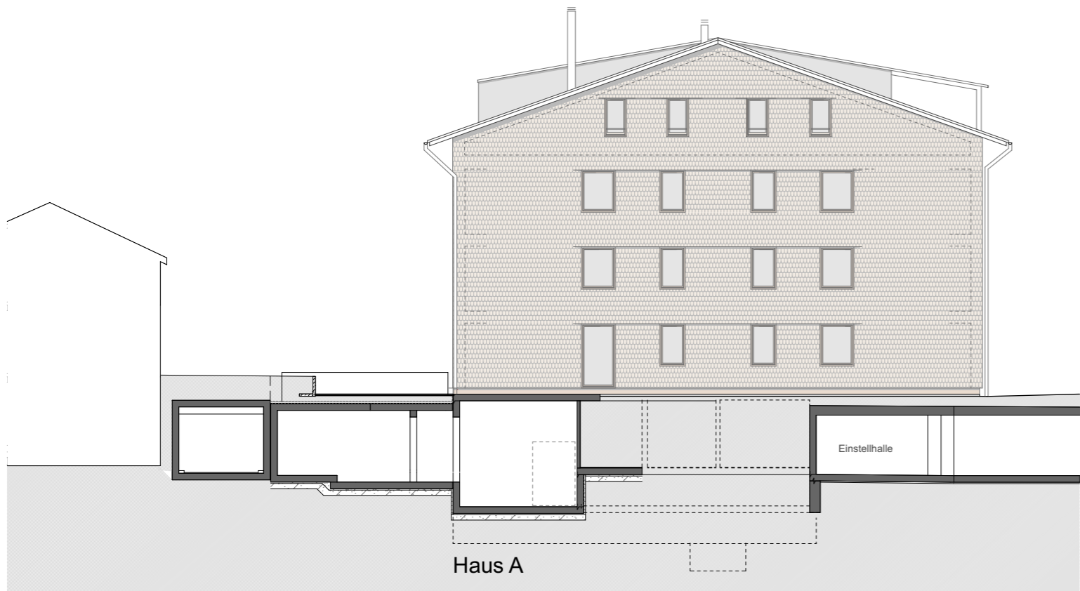
Nordfassade
